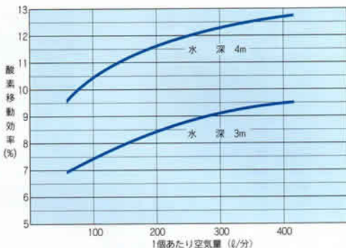
マルチフューザーの酸素移動効率
