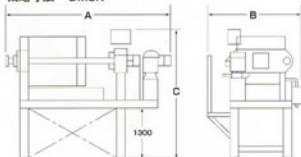
概略寸法 DMSK
