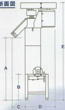
断面図
